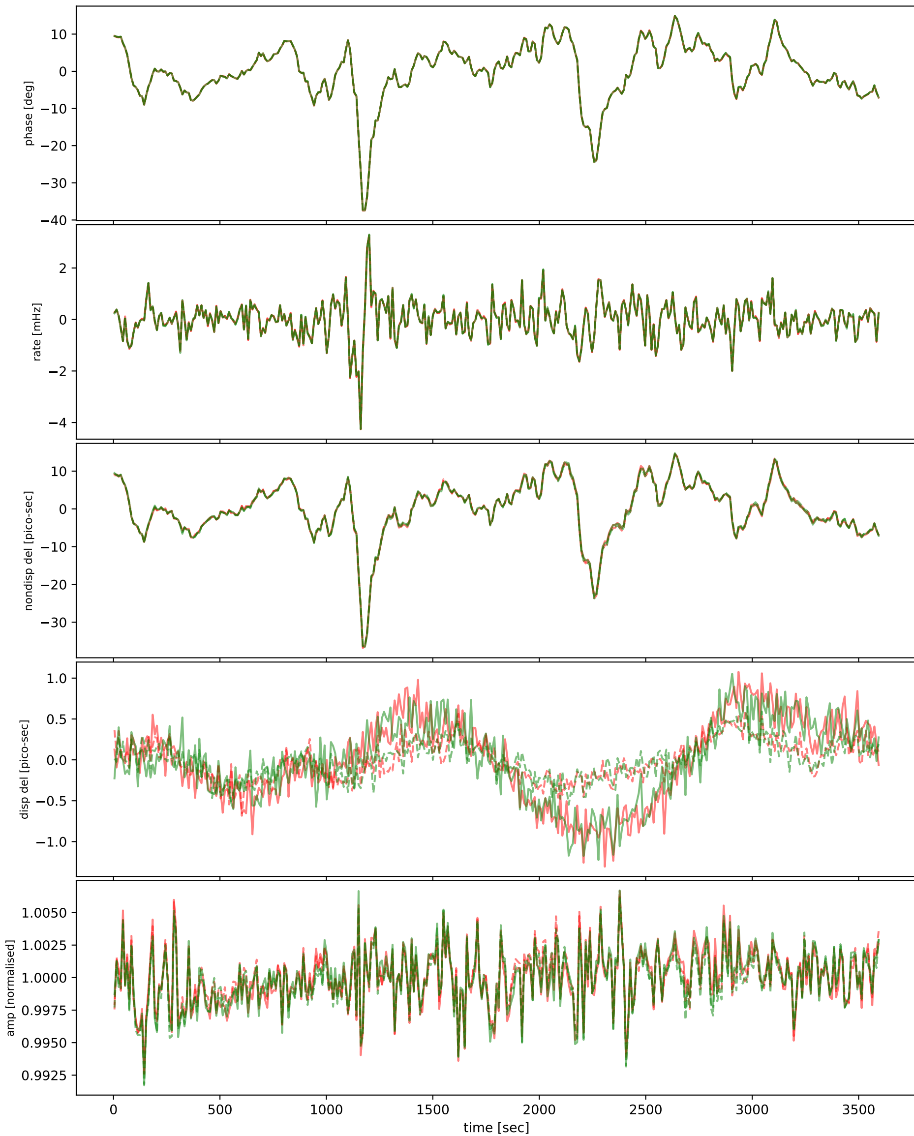
m003-m030
