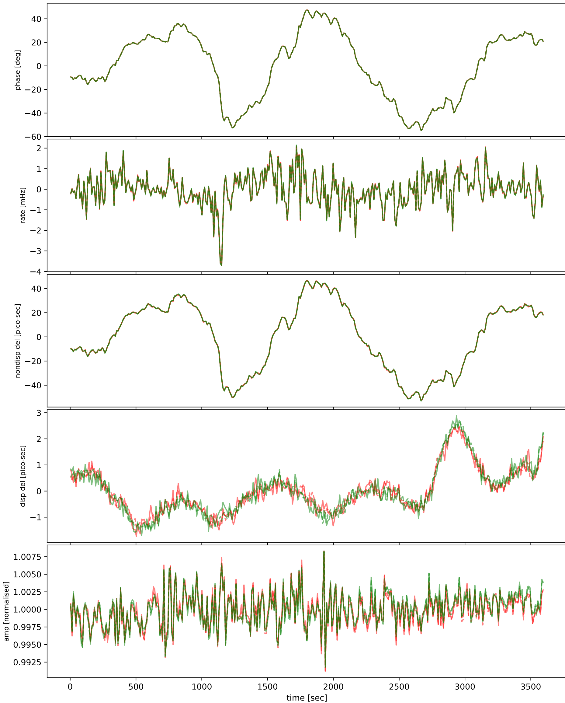
m004-m057
