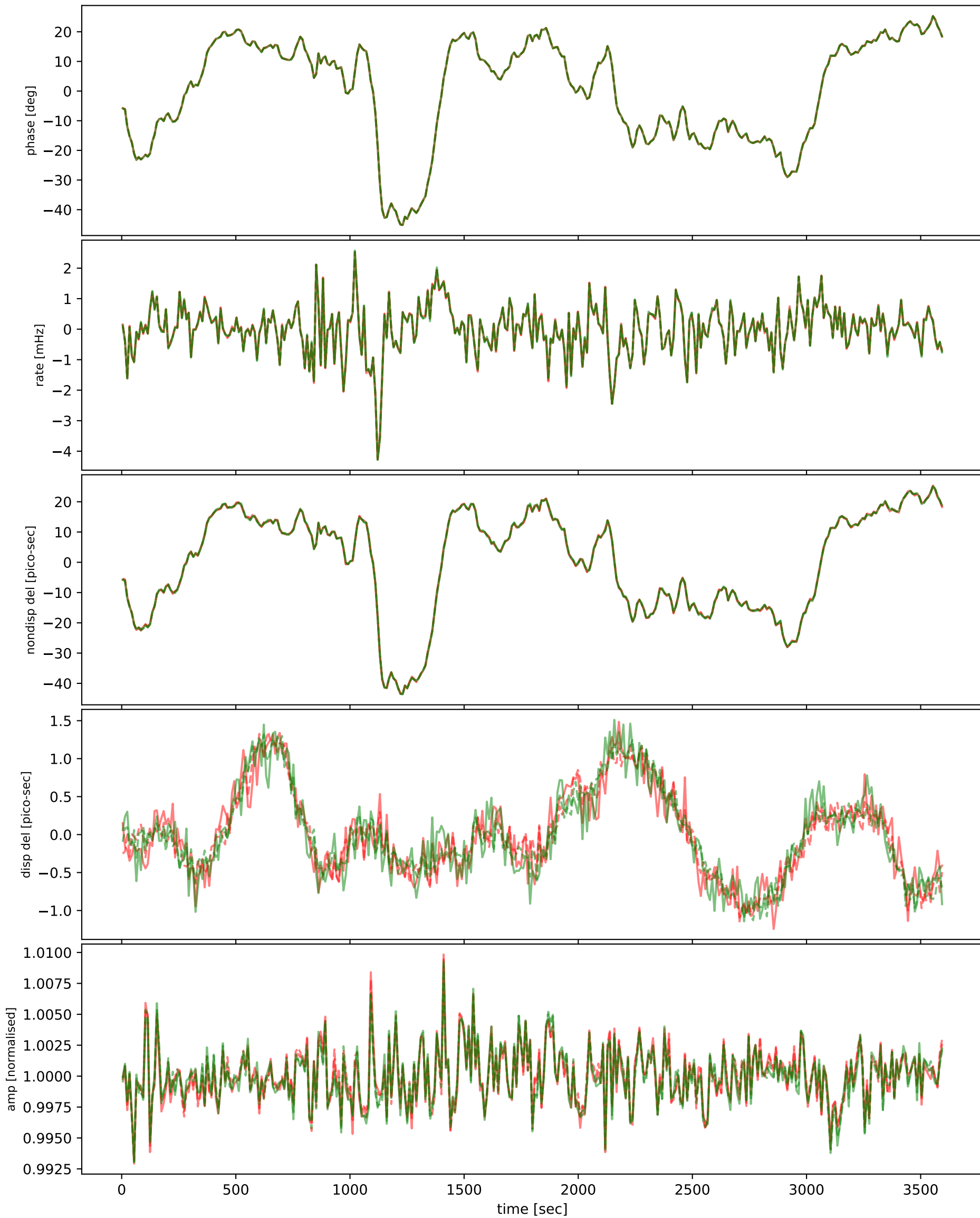
m007-m045
