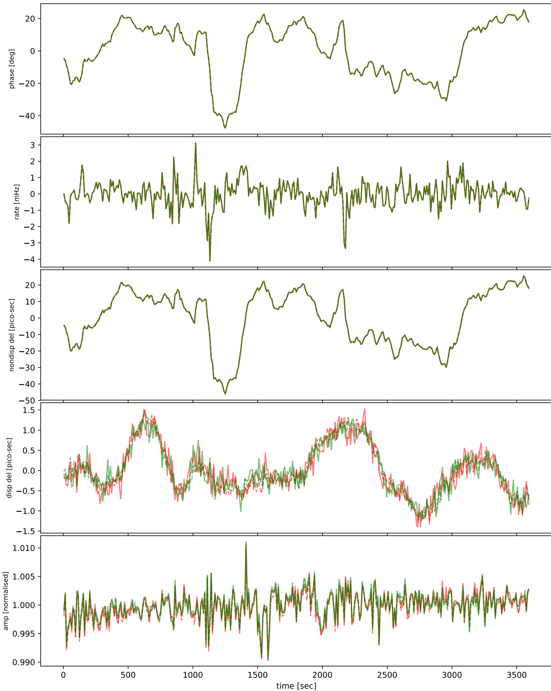
m006-m045
