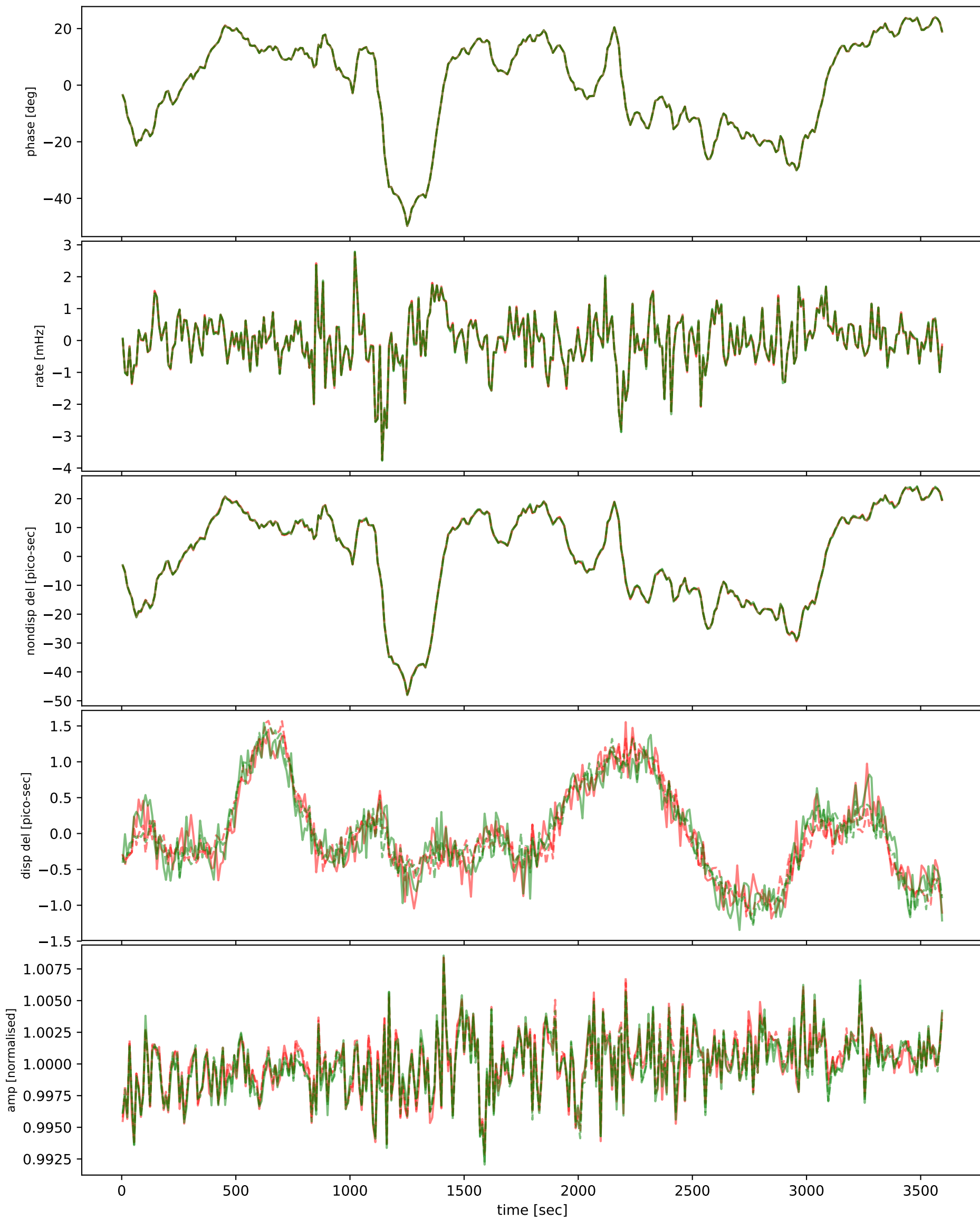
m002-m045
