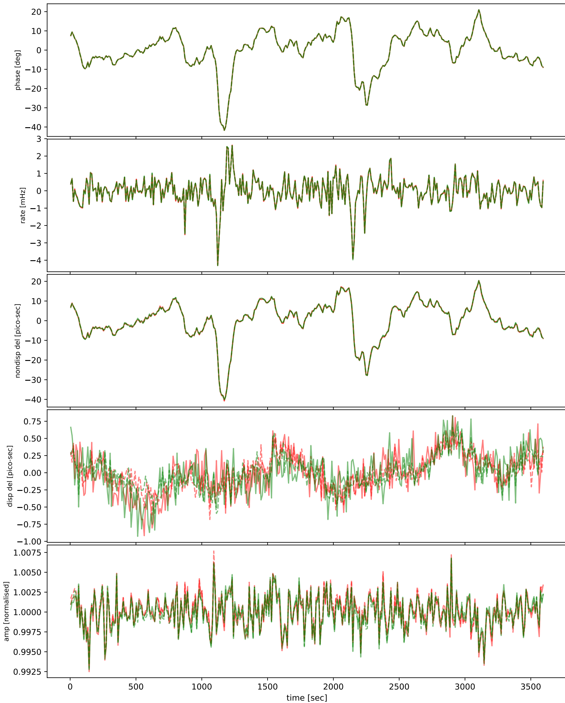
m007-m030
