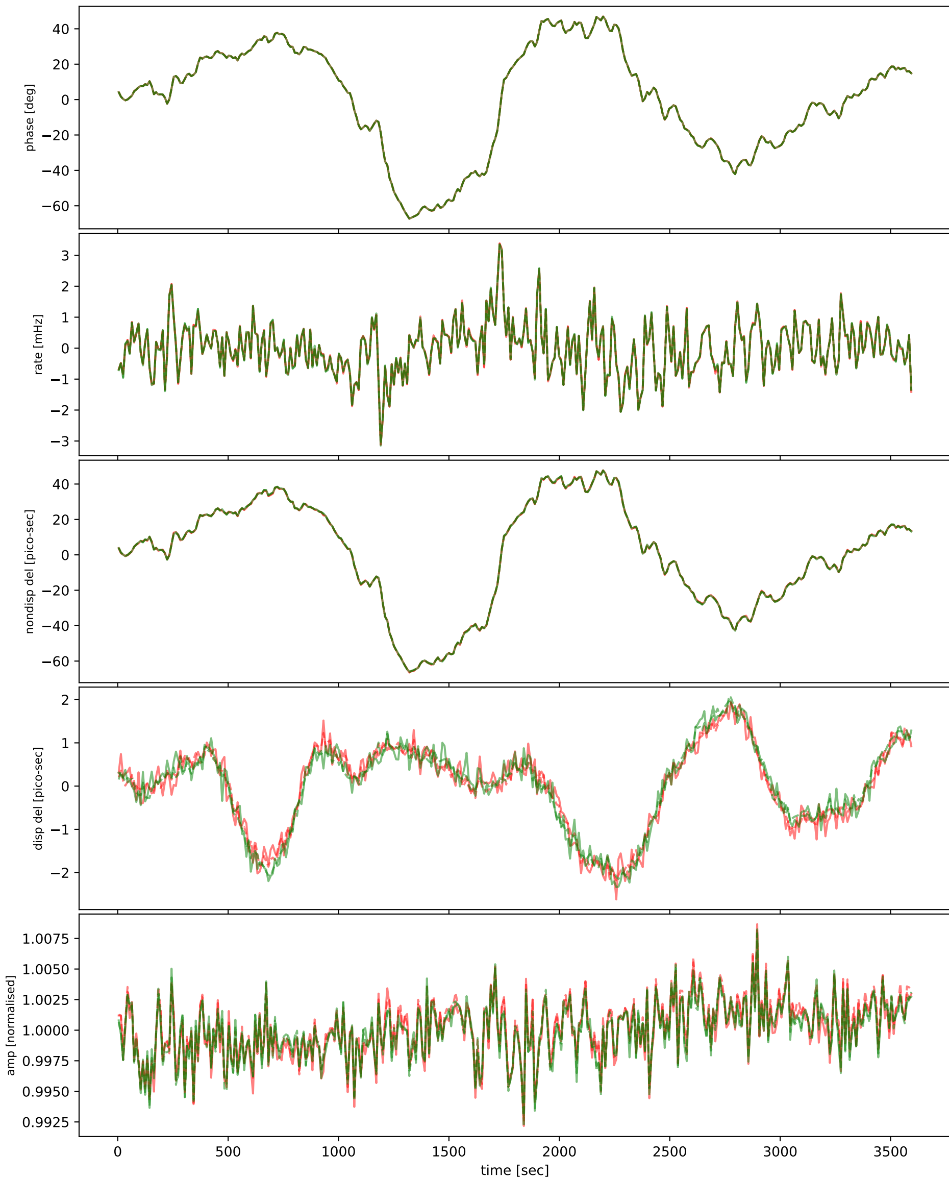
m030-m060
