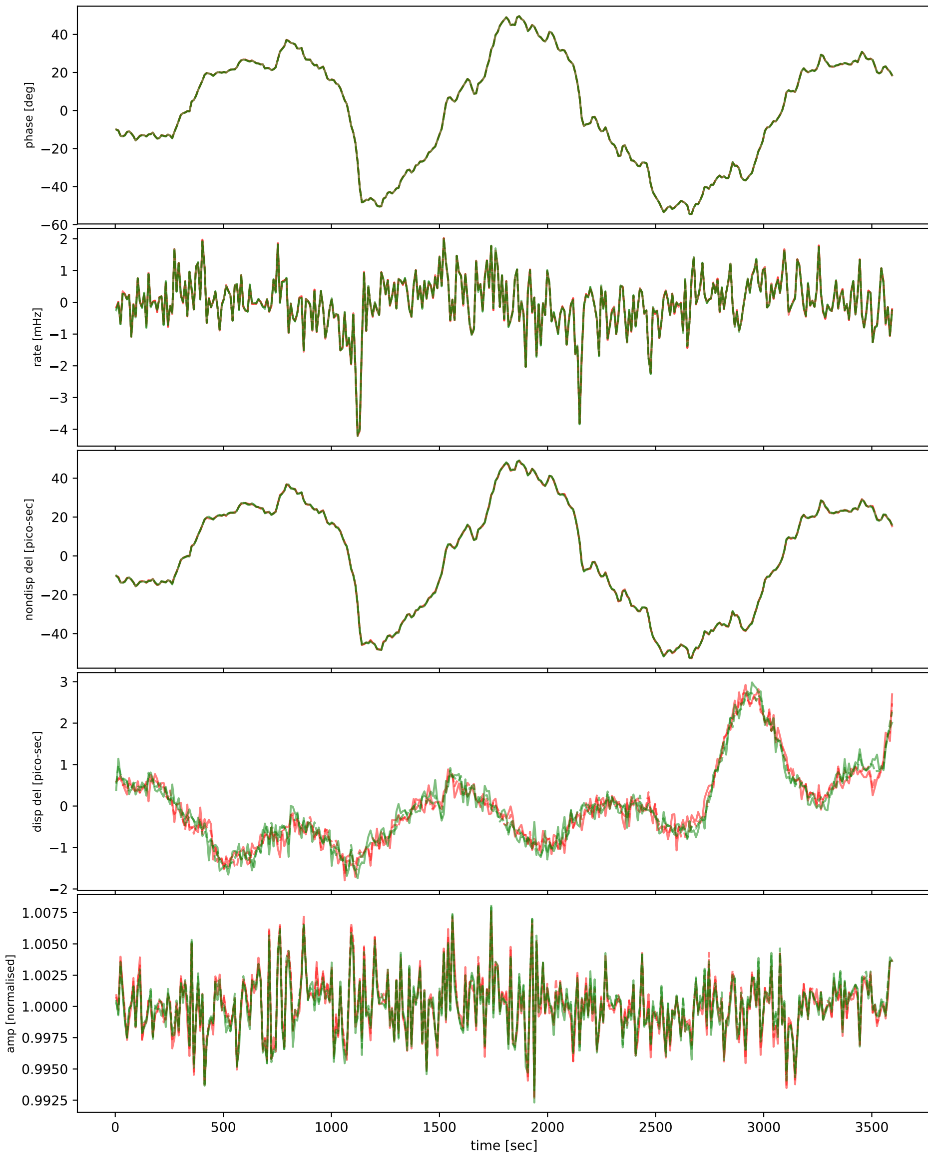
m007-m057
