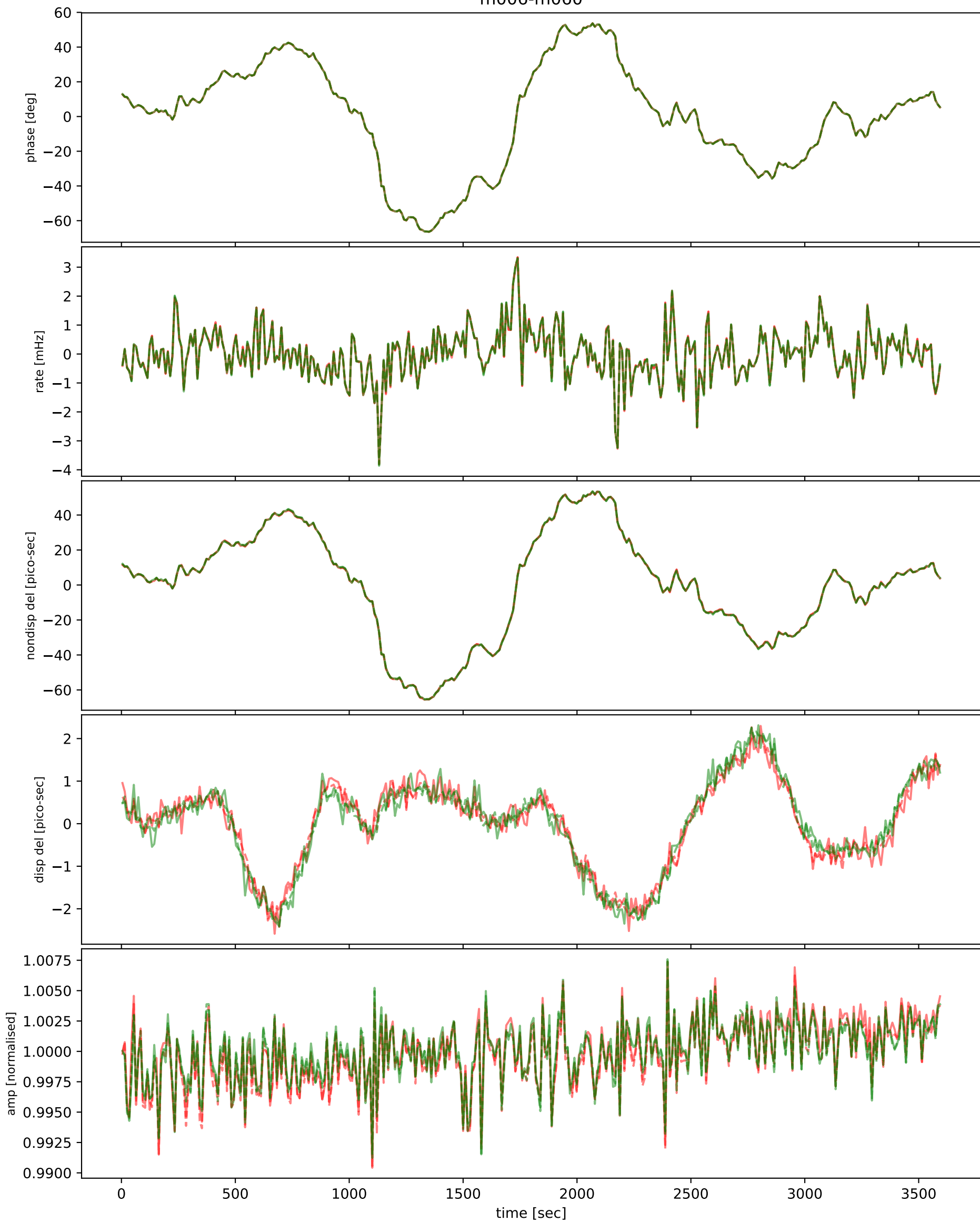
m006-m060
