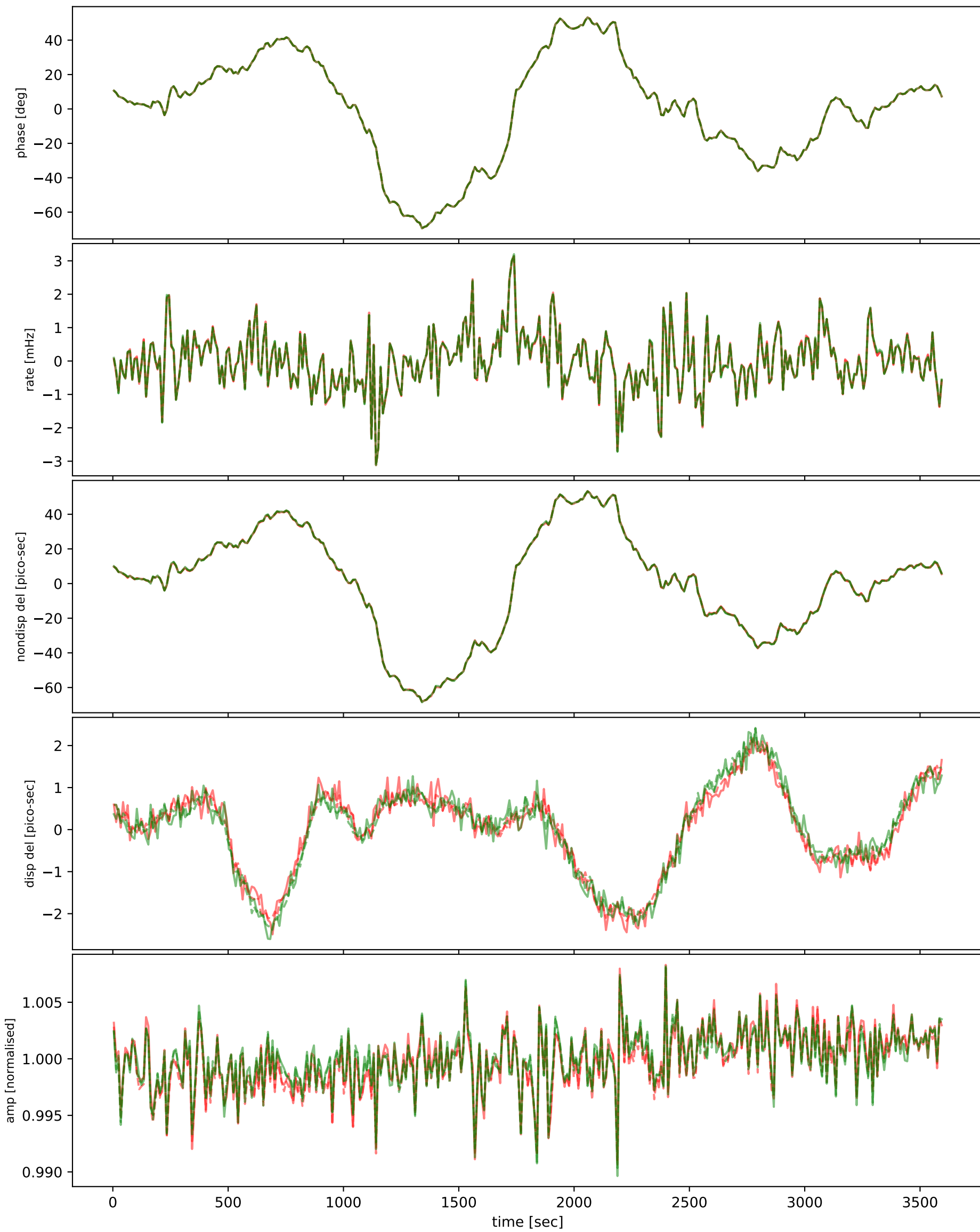
m000-m060
