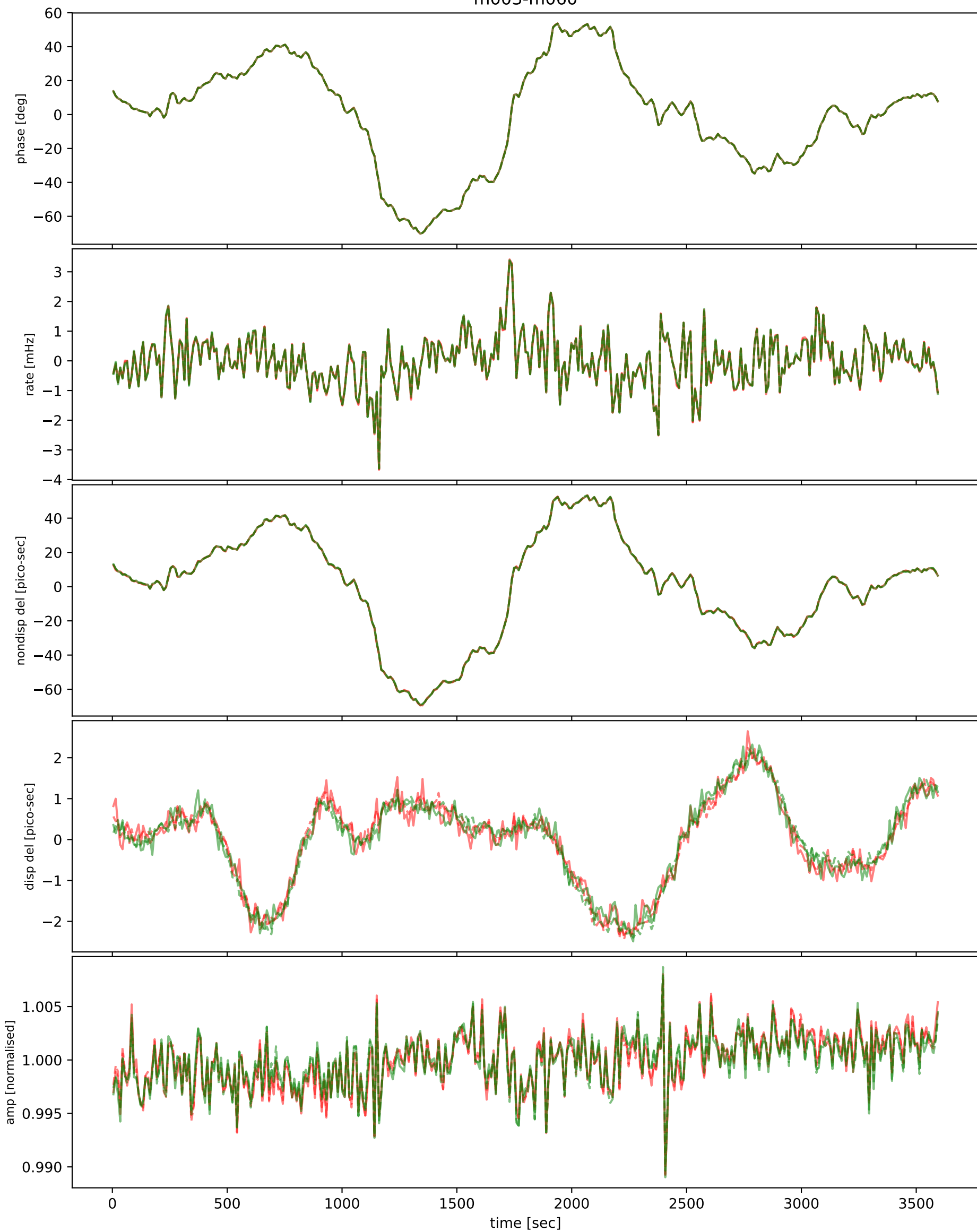
m003-m060
