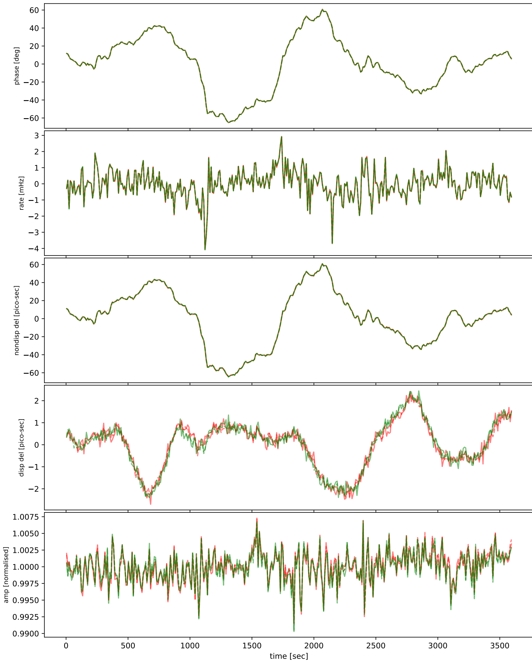
m007-m060
