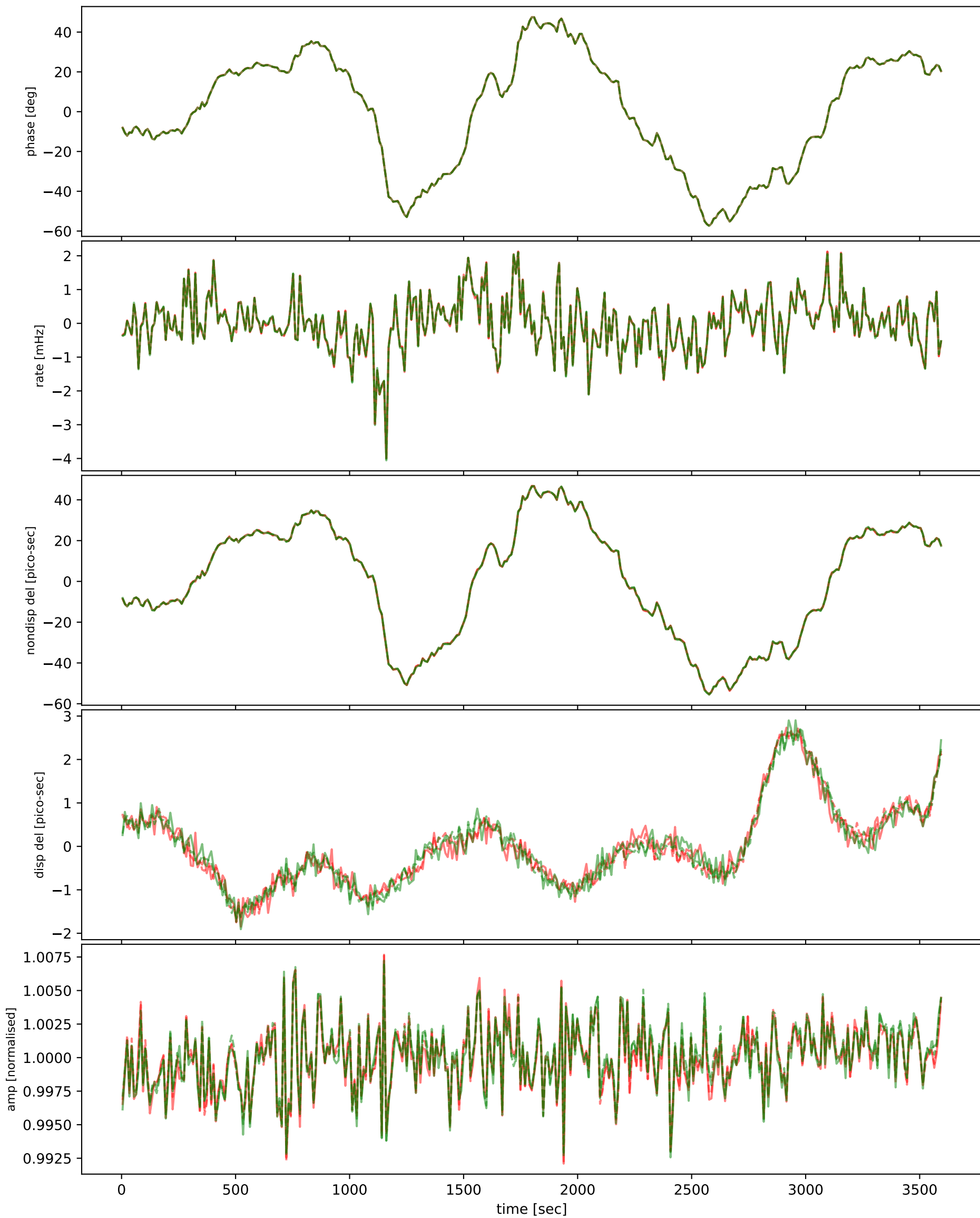
m003-m057
